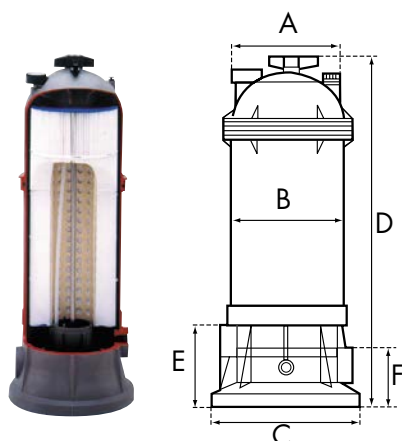
Filtro sección Star Clear™
